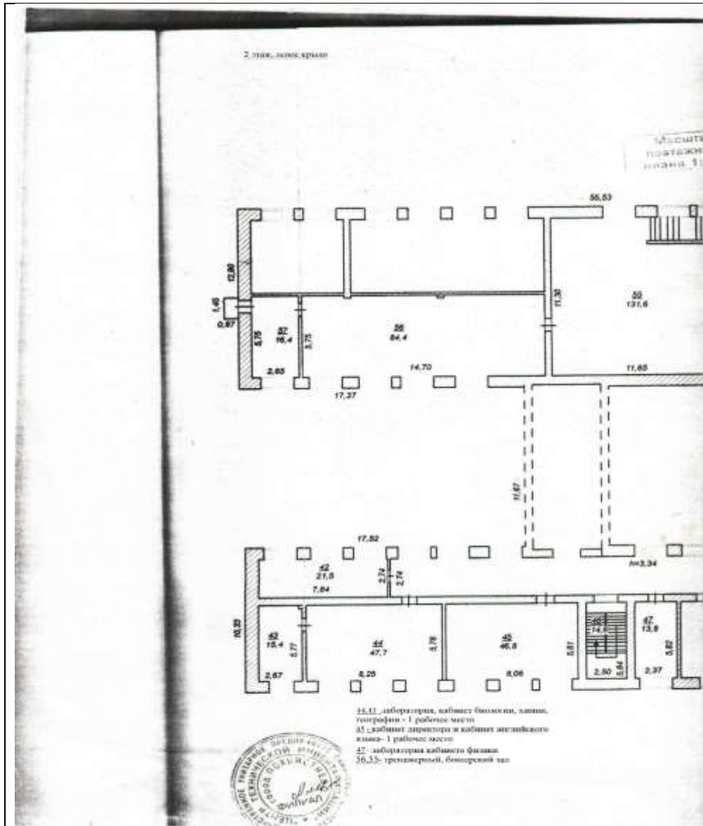
2 этаж
